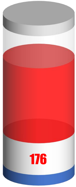
VO Formation
